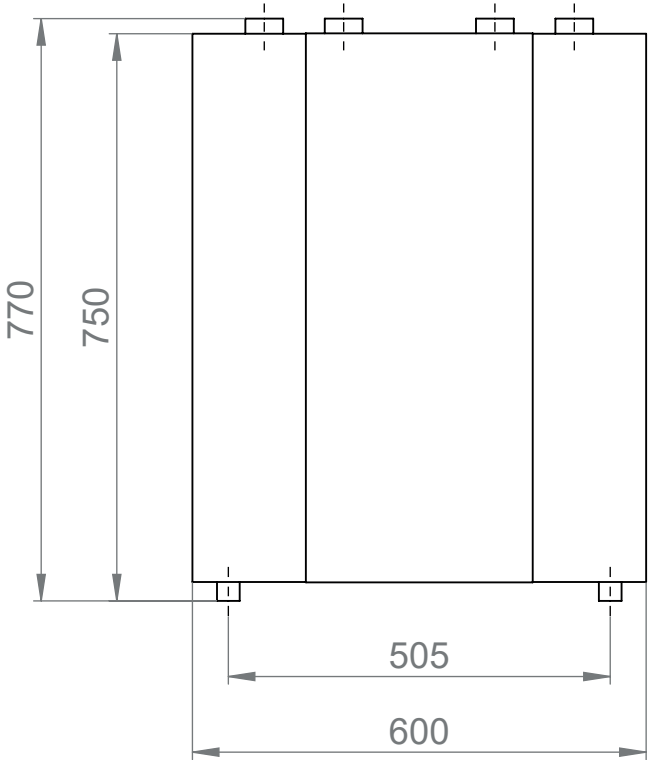
Frontansicht
